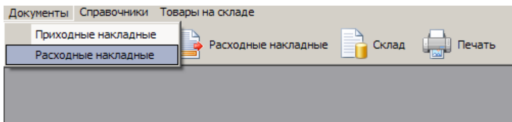
Рисунок 11 - Меню Документы
