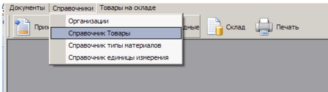
Рисунок 12 - Меню Справочники
