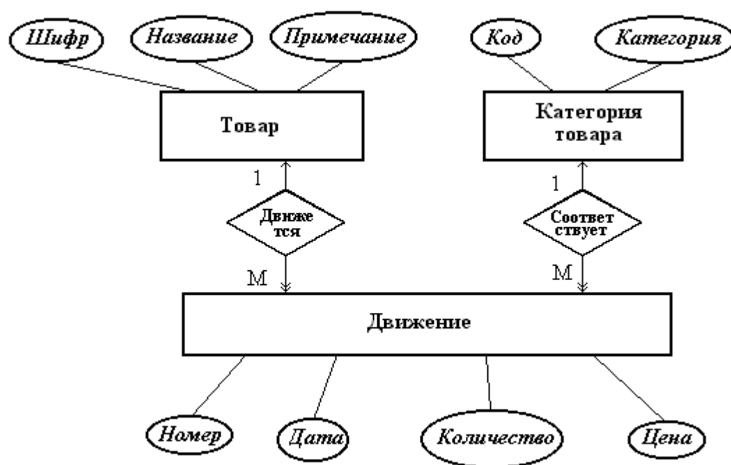
Рисунок 5 - Модель ПО «Движение товара»
