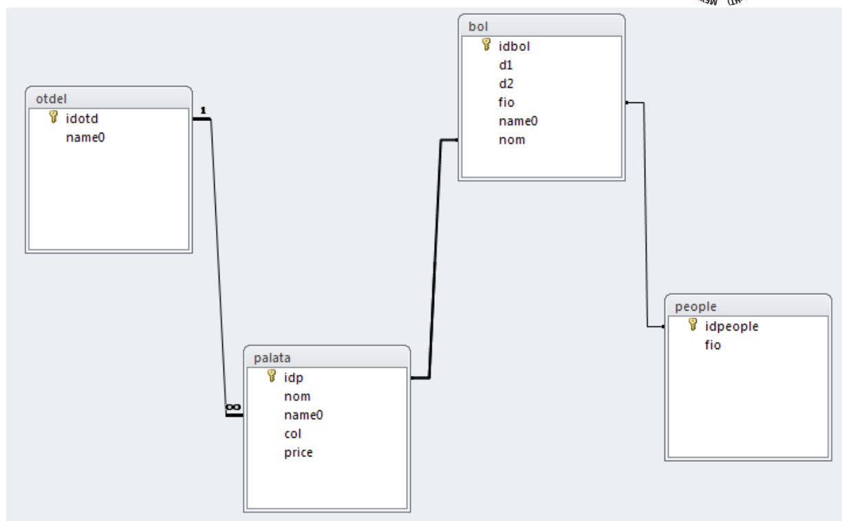
Рисунок 8 - Схема данных предметной области
