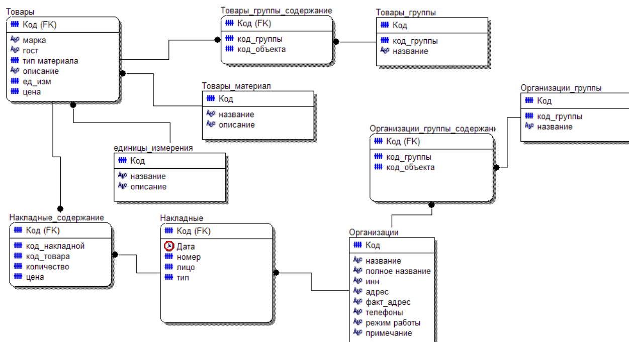
Рисунок 3 - Пример ER диаграммы
