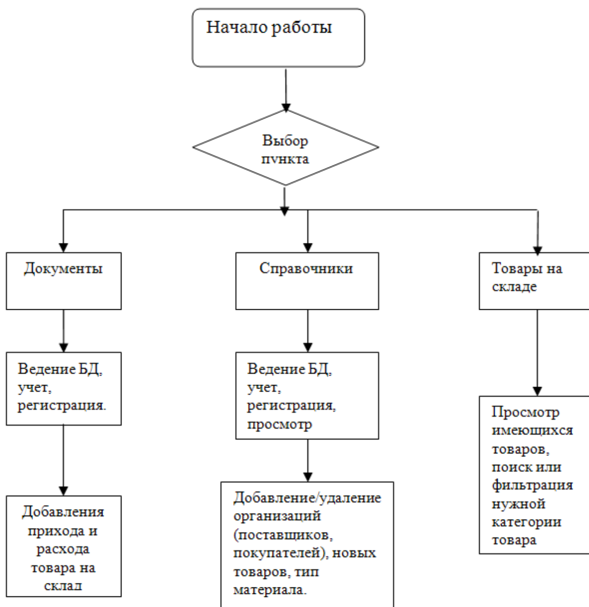
Рисунок 9 - Дерево функций
